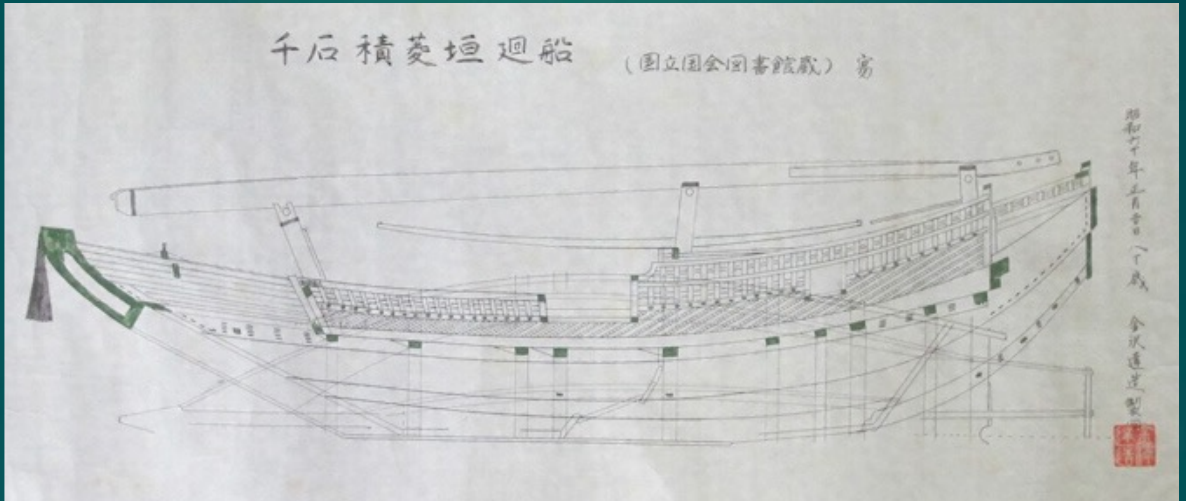
千石積菱垣廻船設計図(模写). 高岡市立博物館 所蔵, 文化遺産オンライン 収録. CC BY. https://jpsearch.go.jp/item/bunka-210424
