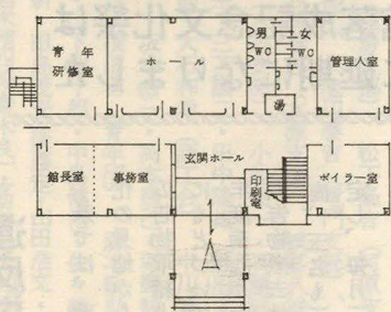
1階平面図
