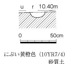
第122図 溝22 (1/30)
