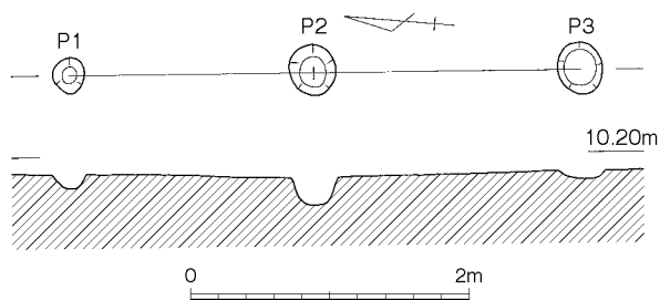
第76図 柱穴列4 (1/60)
