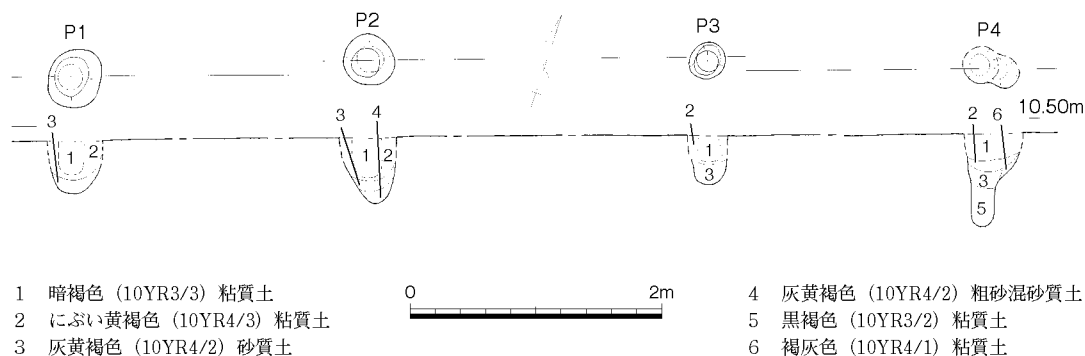
第80図 柱穴列9 (1/60)
