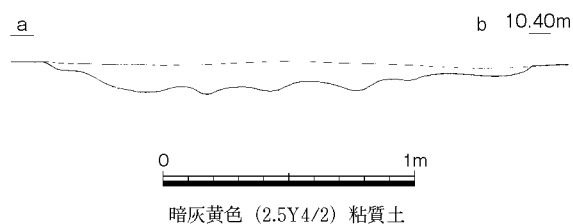
第112図 溝9（1/30）
