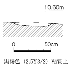
第52図 溝19 (1/30)
