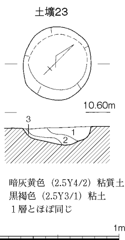
第99図 土壌22～24 (1/30)
