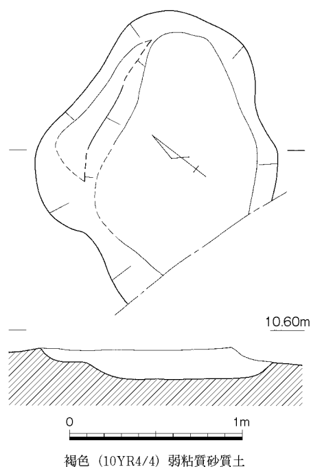
第141図 土壇2 (1/30)
