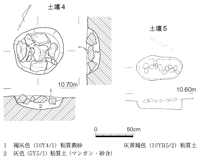
第33図 土壌4・5 (1/30)
