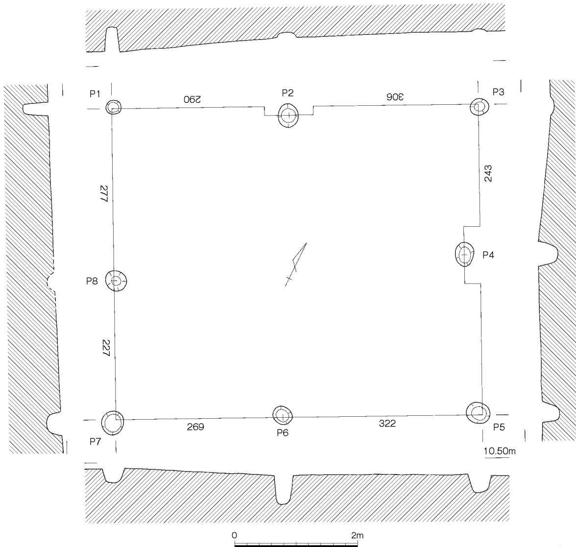
第71図 建物2 (1/60)
