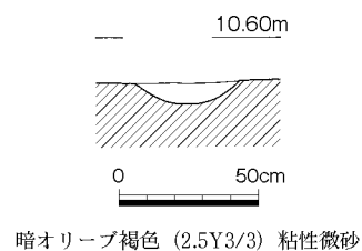
第41図 溝6 (1/30)
