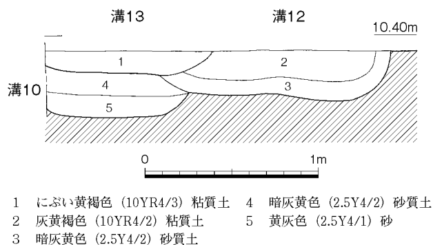
第114図 溝10・12・13 (1/30)
