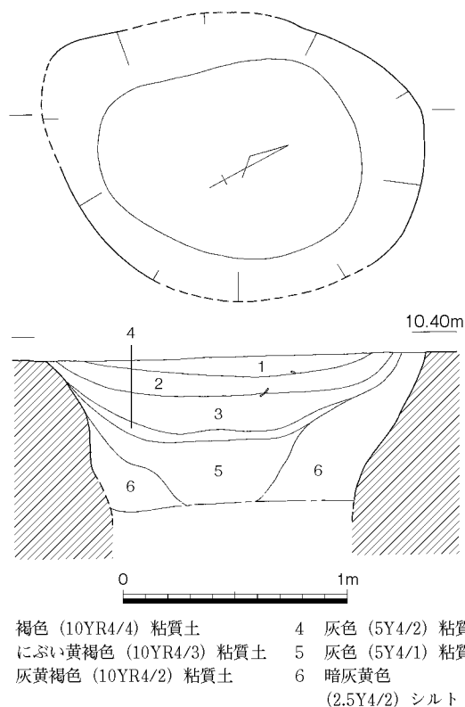
第81図 井戸1 (1/30)
