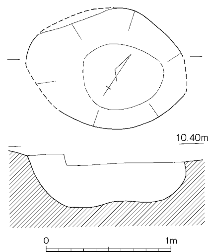
第82図 土壌1 (1/30)
