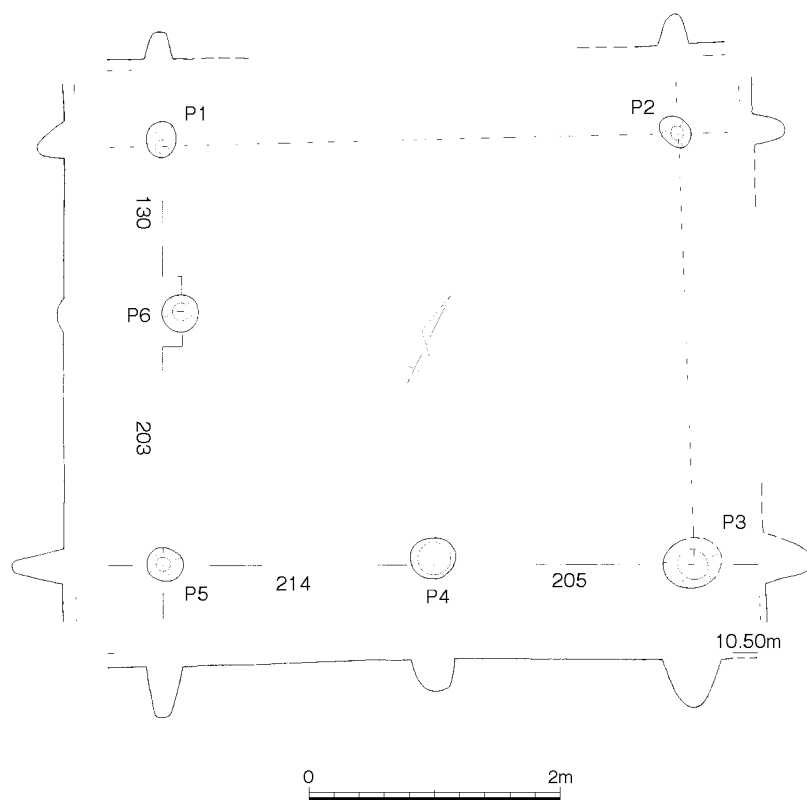
第72図 建物3 (1/60)
