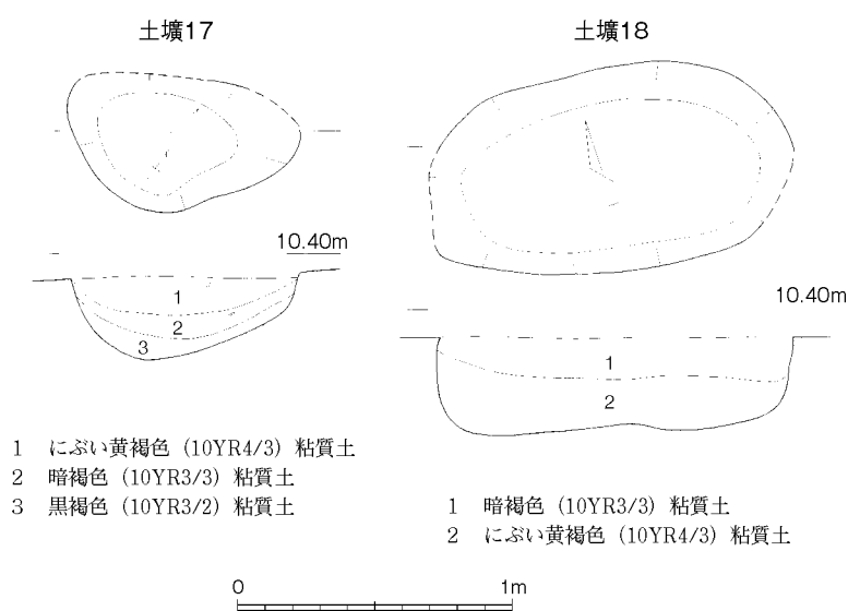
第96図 土壌17・18 (1/30)
