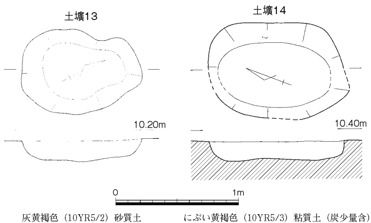
第94図 土壌13・14 (1/30)
