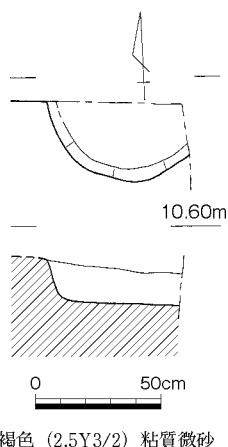
第36図 土壌8 (1/30)
