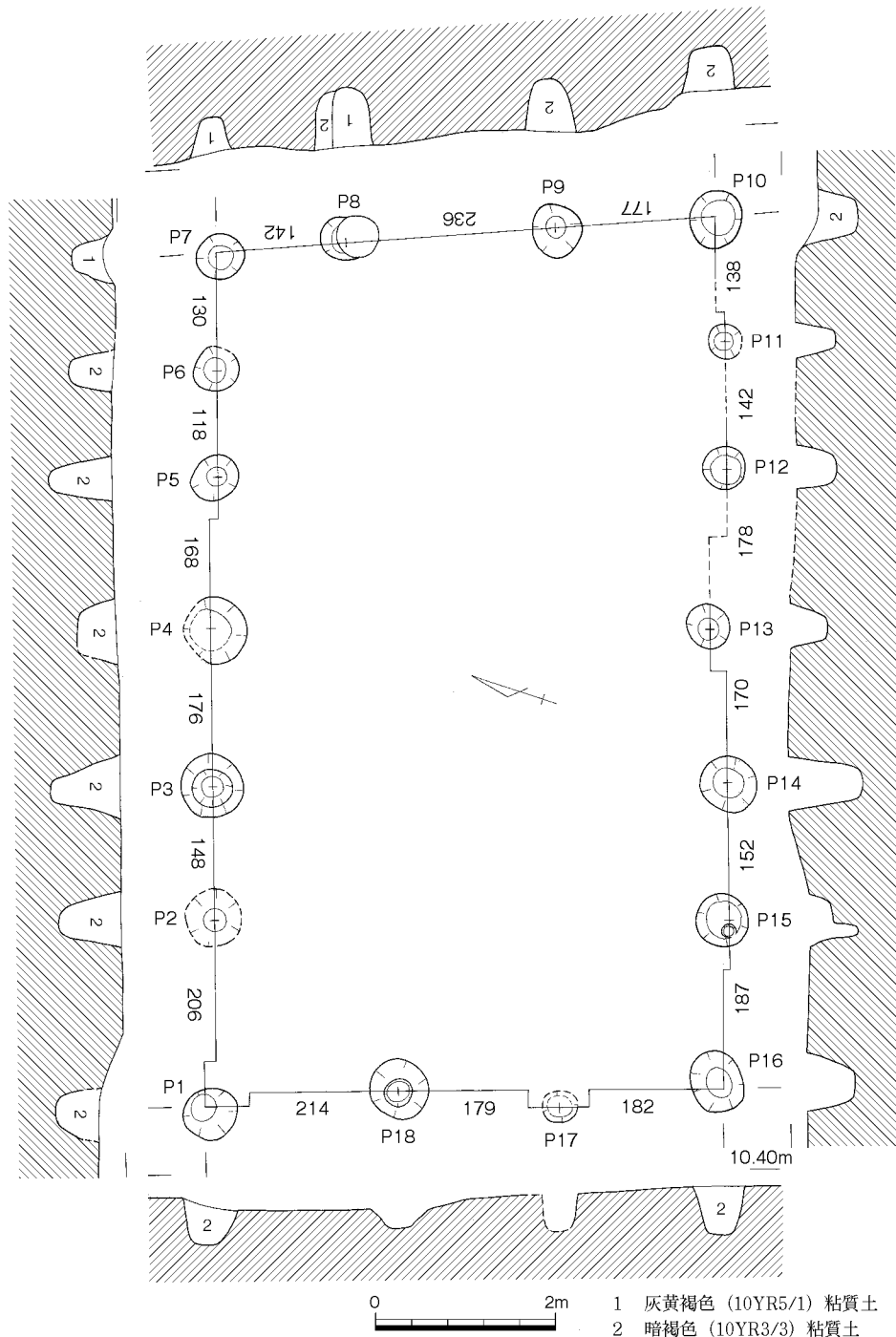
第69図 建物1 (1/80)
