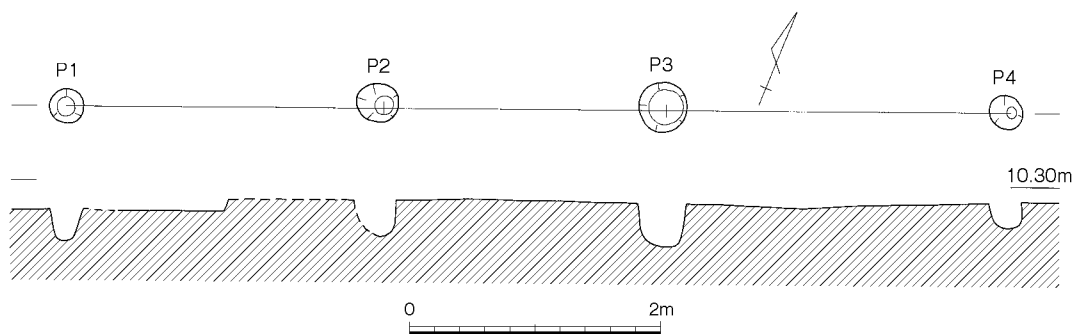
第76図 柱穴列4 (1/60)
