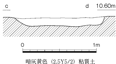
第135図 溝27 (1/30)
