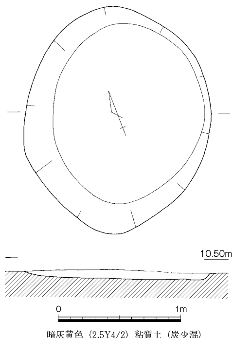
第97図 土壌19 (1/30)
