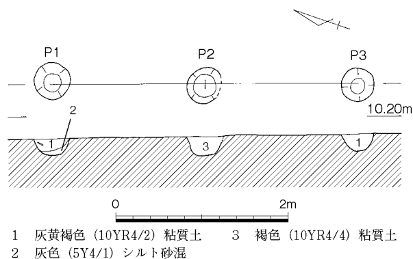
第75図 柱穴列3 (1/60)
