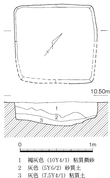
第38図 土壌10 (1/30)
