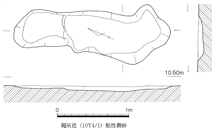
第35図 土壌7 (1/30)
