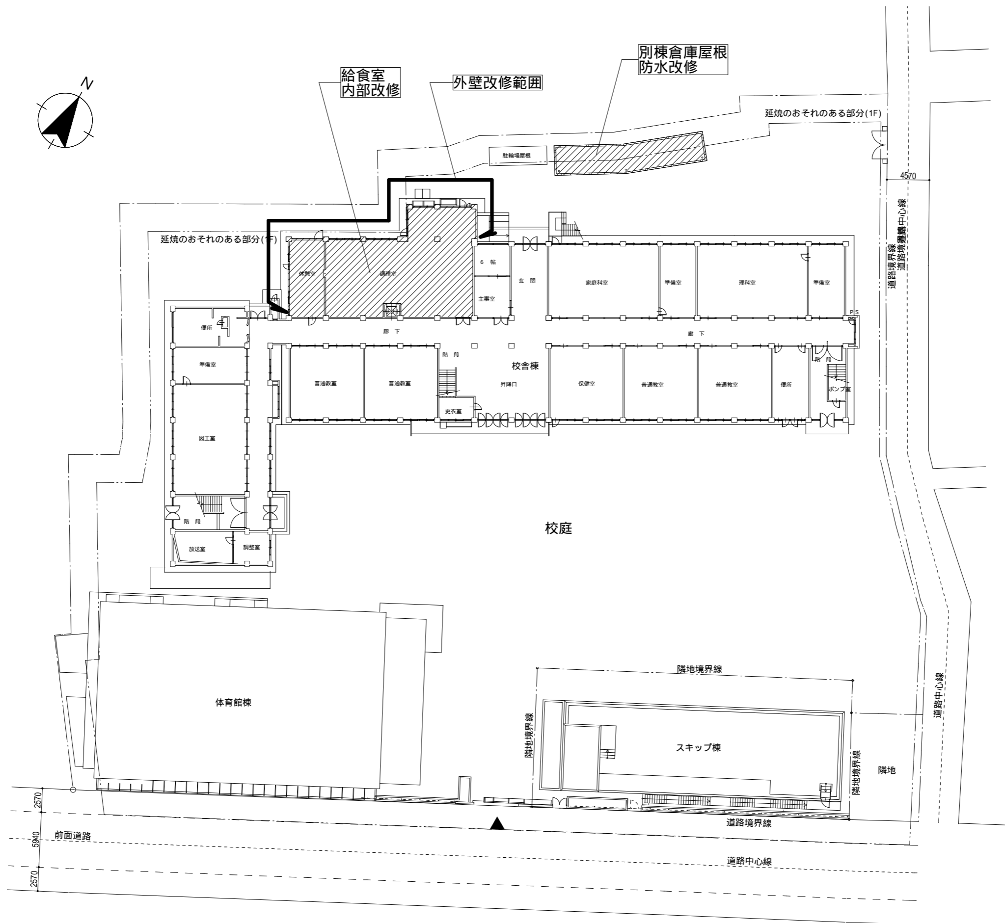
1階平面図兼配置図 S=1/400
